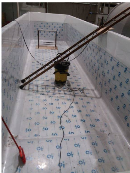
Tanques em aço revestidos com placas em PVDF com tecido
